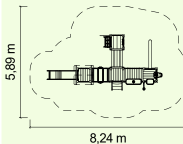
Grundriss: 1:200
