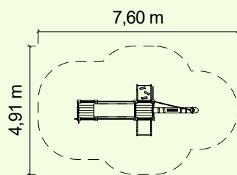
Grundriss: 1:200
