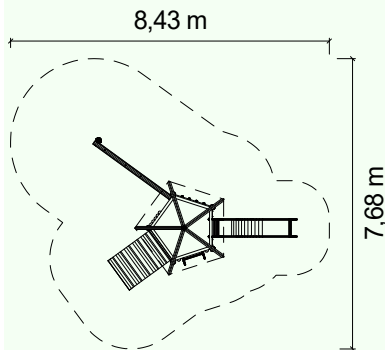
Grundriss: 1:200
