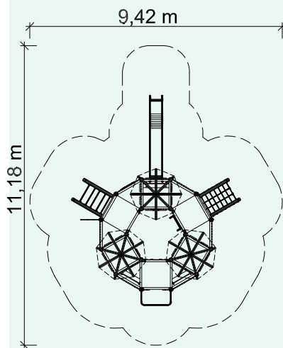
Grundriss: 1:200
