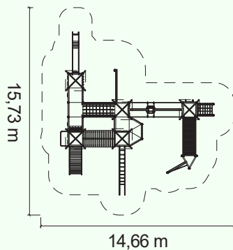
Grundriss: 1:400
