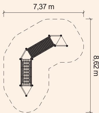
Grundriss 1:200
