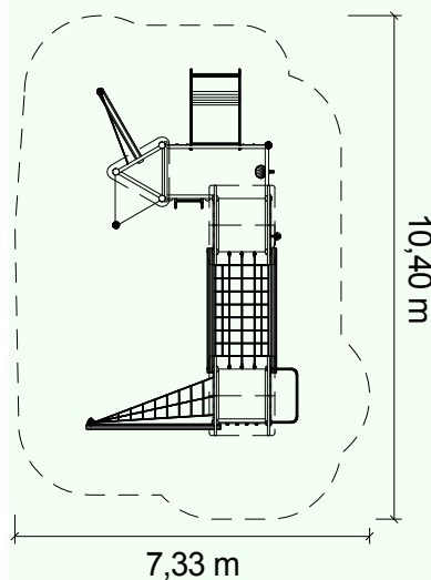
Grundriss: 1:200
