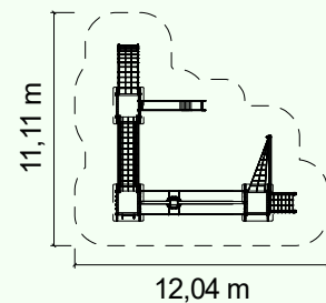
Grundriss: 1:400
