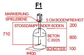
Stoßdämpfender Boden nach DIN 1176 (Tabelle siehe Wartungsanleitung)
