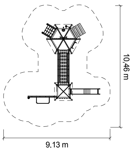
Grundriss: 1:200
