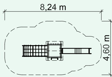
Grundriss: 1:200
