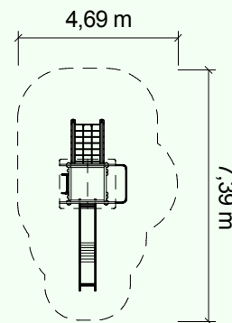
Grundriss: 1:200
