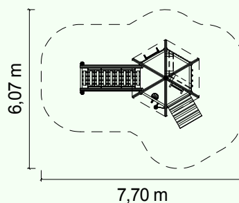
Grundriss: 1:200
