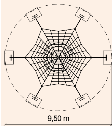
Grundriss 1:200
