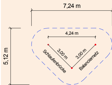
Grundriss 1:200
