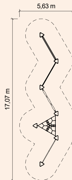
Grundriss 1:200
