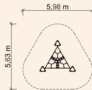
Grundriss 1:200
