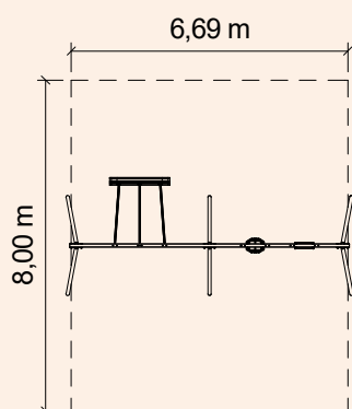
Grundriss 1:200
