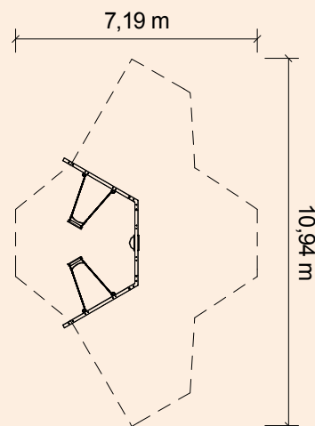
Grundriss: 1:200
