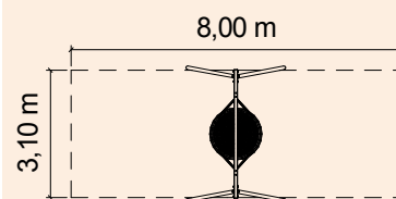
Grundrisse: 1:200
