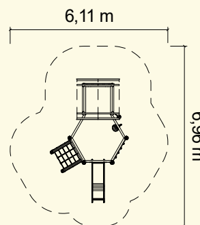
Grundriss: 1:200
