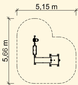
Grundriss: 1:200
